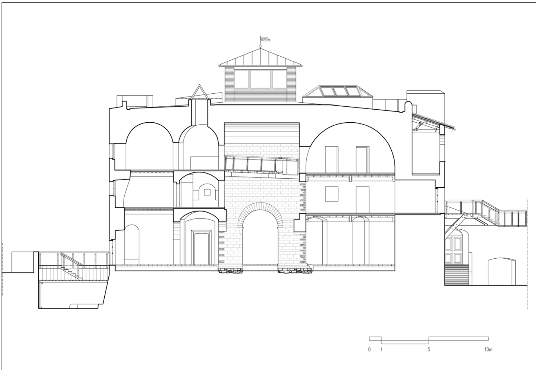
Sezione longitudinale dopo il restauro
