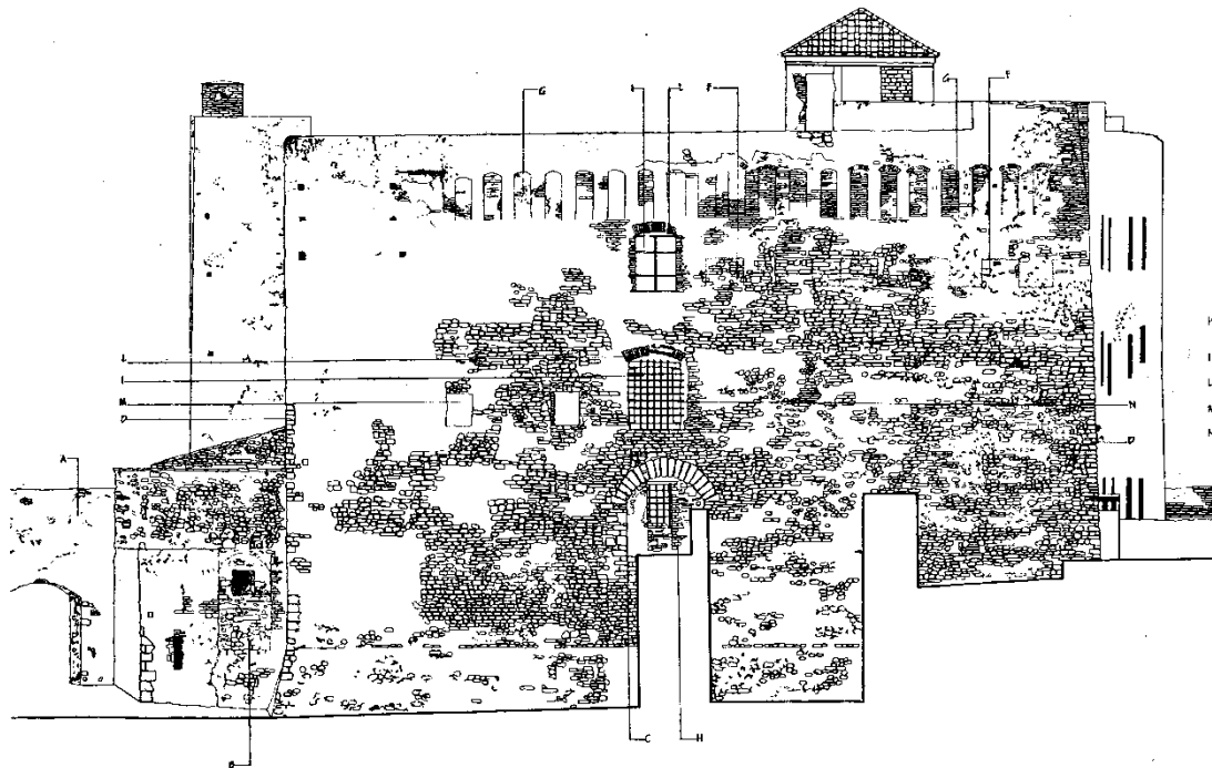
Prospetto ovest - Rilievo
