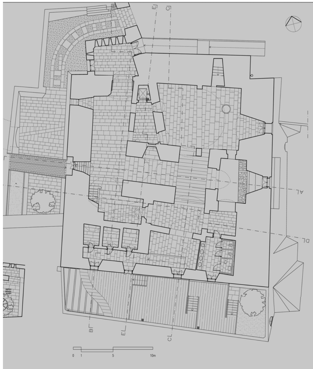
Progetto – pianta piano terra
