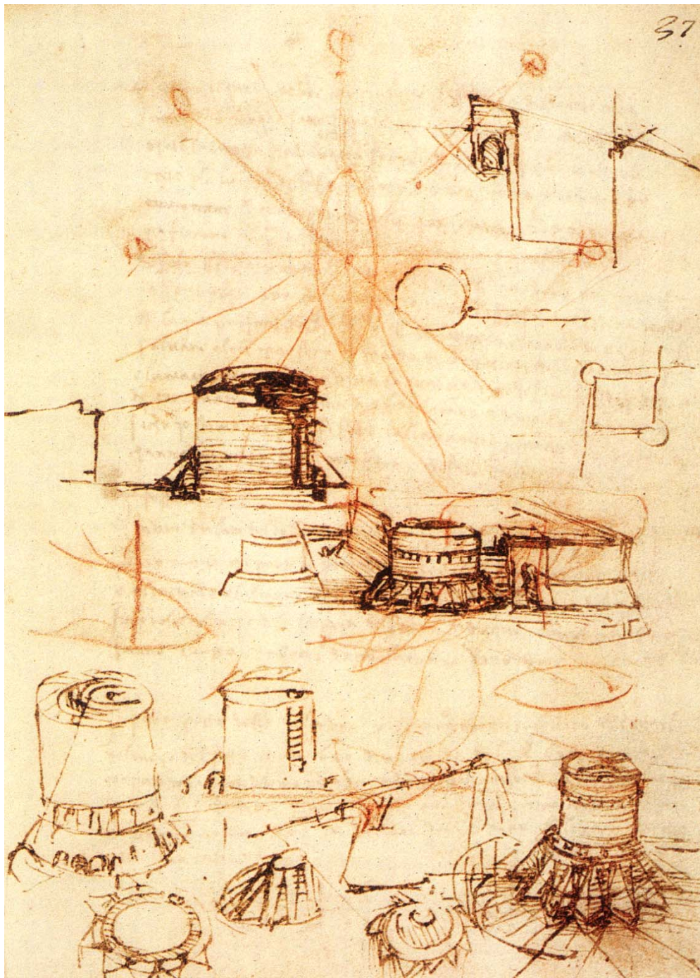
Leonardo. Da Vinci – Progetto per un bastione circolare nel castello di Piombino (1502 c.) – Codice di Madrid II, 37r
